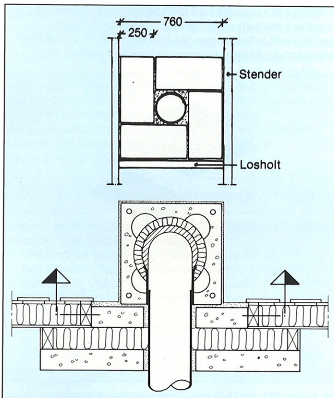
Fig. 10. Leca pipe kan monteres utvendig uten tilleggsisolasjon. Røykrør føres gjennom vegg og omsluttet med LECA blokker som gir forskriftsmessig avstand til treverk (230 mm). Innvendig 100 mm Leca blokk som brannmur.
