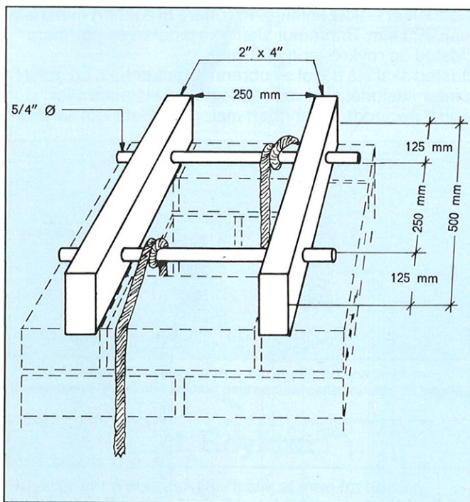
Fig. 21. Bremsegrind.
