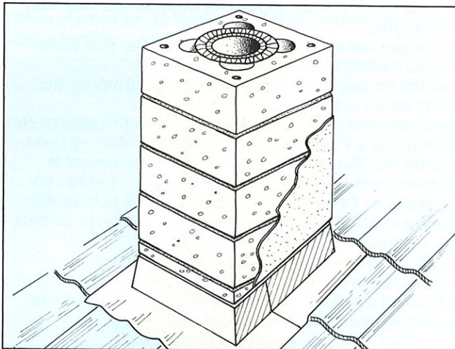
Fig. 13. Type PBF er et beslag med formbar fot av bly tilpasset krum takstein (f.eks. Zanda) eller lignende tekkematerialer. Beslaget kan kun benyttes på pusset Leca ettløps pipe.
