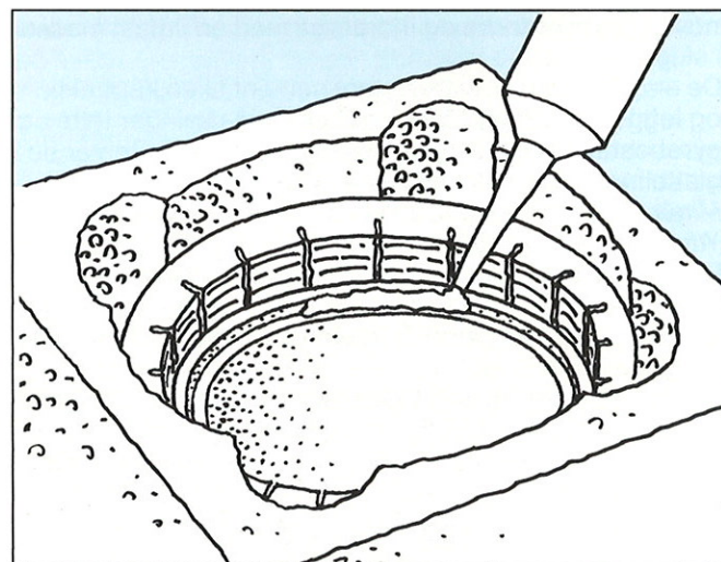
Fig. 7. Ildfast masse påføres foringsenden.
