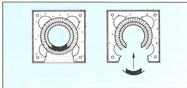
Fig. 18. Plassering av igjenmuringslokk.
