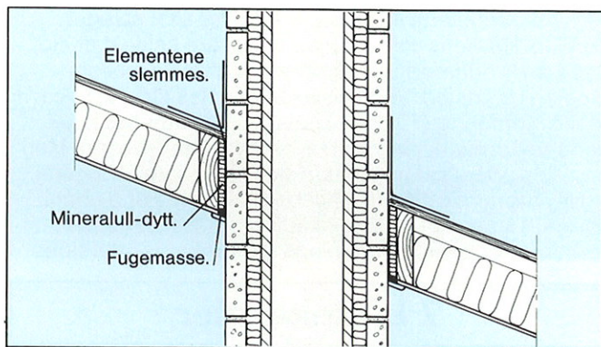
Fig. 9. Gjennom loftsbjelkelag eller isolert takkonstruksjon anbefales at ytterelementene ved gjennomgangen mørtelslemmes utvendig før montering. Spalten mellom ytterelement og trebjelker dyttes med mineralull og forsegles fra undersiden med elastisk fugemasse.
