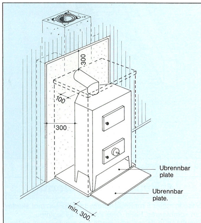
Fig. 25. Lukket ildsted.
