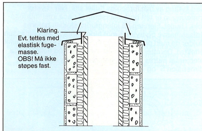
Fig. 11. Toppbeslag og pipehatt i aluminium leveres til så vel ettløps som toløps Leca pipe. Toppbeslag må forankres godt. Monteringsveiledning i kartongene. Ønskes annen utforming av toppen, kan dette gjøres f.eks. med en på plassen støpt betonghelle. Husk at pipeforingen må ha anledning til å "arbeide" uten å støte mot topplaten.
