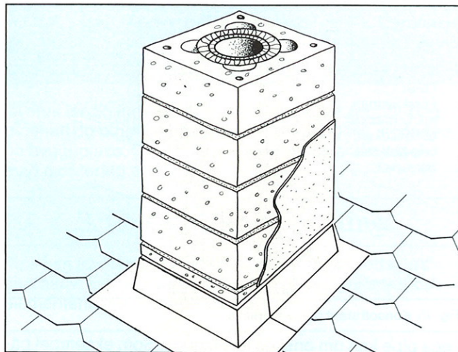
Fig. 12. Type PB er tilpasset for flatt takbelegg (papp, shingel m.m.). Dette beslaget er teleskopisk i to retninger og kan anvendes på ettløps og toløps pusset pipe.
