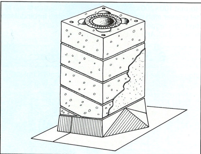
Fig. 14. Høye piper over tak kan avstives mot vindbelastning ved å armere og istøpe hjørnehullene. Dersom pipa er plassert langt nede på taket, bør en piperygg anordnes som snøavviser (lages på stedet) eller snøfangere monteres på oppsiden av pipa.
