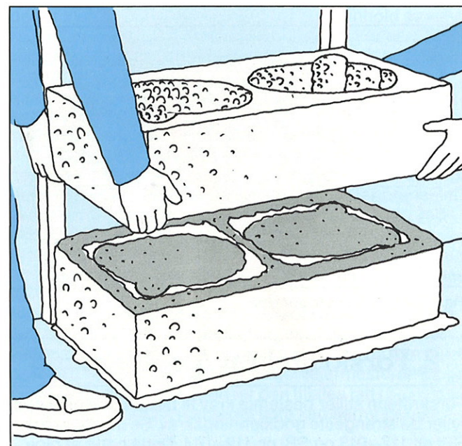
Fig. 8. Toløps pipe mures på tilsvarende måte som ettløps pipe. To mann er mest praktisk til muring av toløps pipe.
