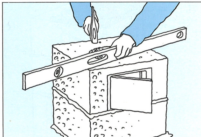
Fig. 2. Hele fundamentet dekkes rikelig med mørtel og første element settes på plass og vattres nøyaktig. For å oppnå tett kjerne under feieluke, fylles utsparring i sokkelement med ubrennbart materiale (sand e.l.) og avrettes med mørtel. Bunnen i feielukeelement tildannes med mørtel – fall innover fra åpningen.
