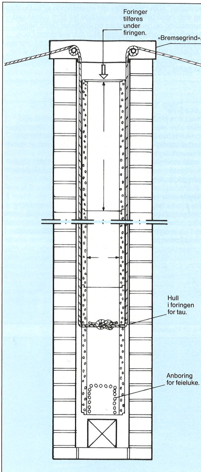
Fig. 22. Vertikalsnitt.
