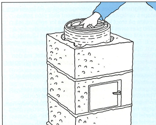
Fig. 4. Mineralull skyves ned med monteringslokket.
