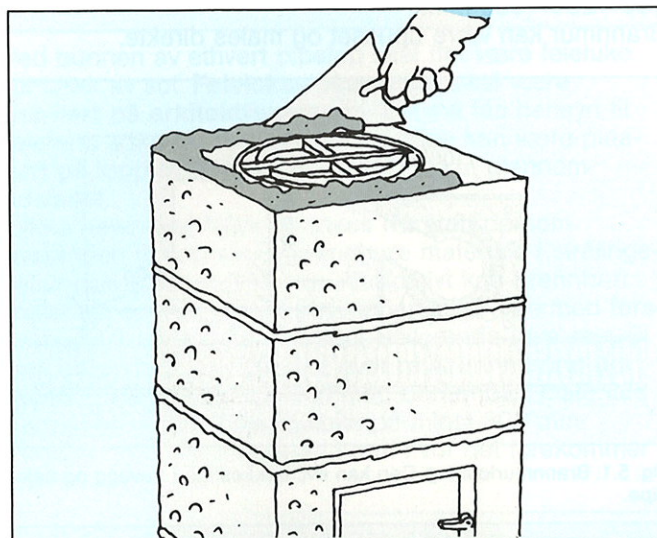
Fig. 1.3. Legg mørtelen godt ut langs ytterkanten under muringen, slik at ikke mørtel presses innover. Monteringslokket blir liggende på mineralullen for å oppta mørtelspill fra den videre muring. Mørtelforbruk, ca. 3 lm pipe pr. sekk Leca Murmørtel (25 kg).
