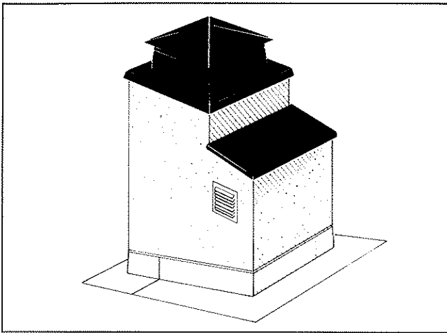
Fig. 2.4. Luftekanal avsluttes et skift under topp skorsteinsløp - dekket med en skiferhelle e.l. 6" ventil i hver side.
