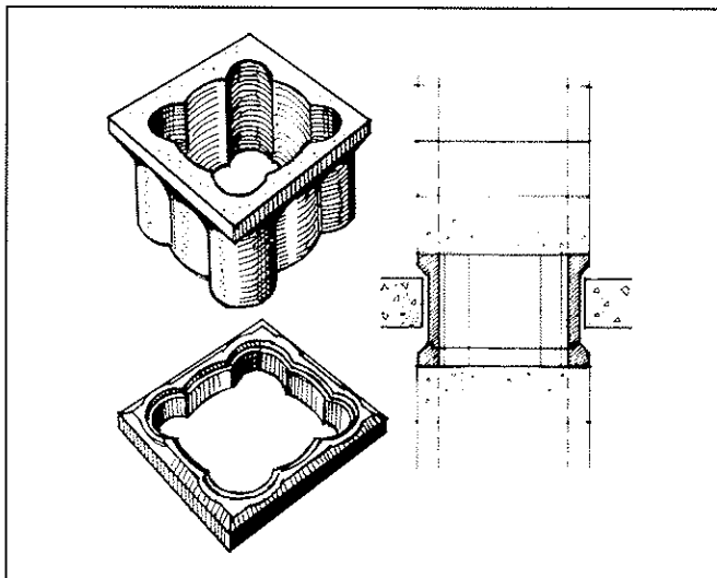
Fig. 7.1. Spesialelement for gjennomføring i støpt dekke.
