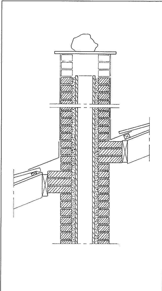
Fig. 3.1. Isolering.
