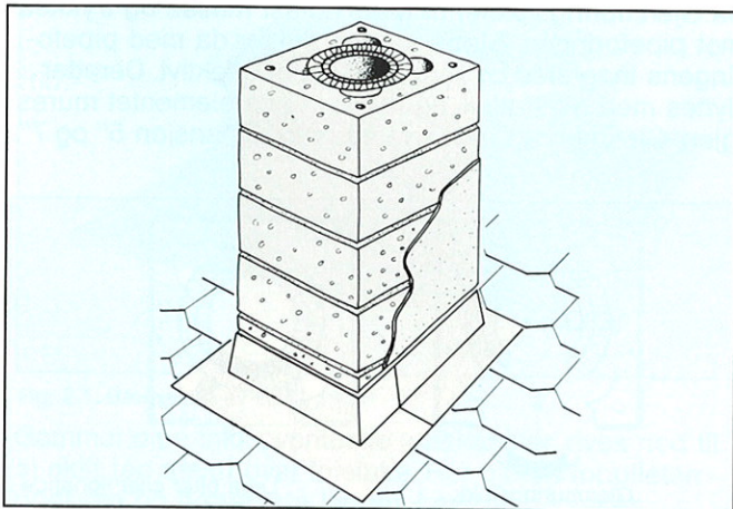
Fig. 1.7. Type PB er tilpasset for flatt takbelegg (papp, shingel m.m.). Anvendes på ettløps pusset pipe.
