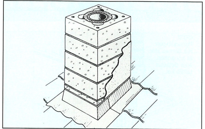
Fig. 1.8. Type PBF (for ettløps) og DPB (for toløps) er beslag med formbar fot av bly tilpasset krum takstein (f.eks. Zanda) eller lignende tekkematerialer.
