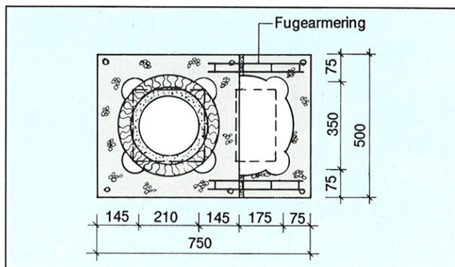
Fig. 2.3. Leca Pipe i kolonne med luftpipe av halve Leca pipeelementer fra loft.
