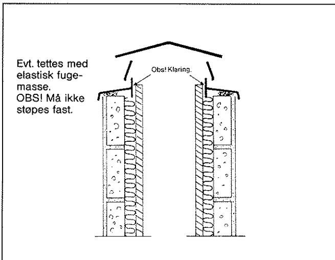
Fig. 3.1. Toppbeslag og Pipehatt i aluminium leveres til så vel ettløps som toløps Leca Pipe. Toppbeslag må forankres godt. Monteringsveiledning i kartongene.
