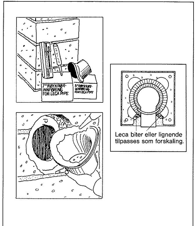
Fig. 4.1. Montering av røykrørrinnføring. Meget viktig.
