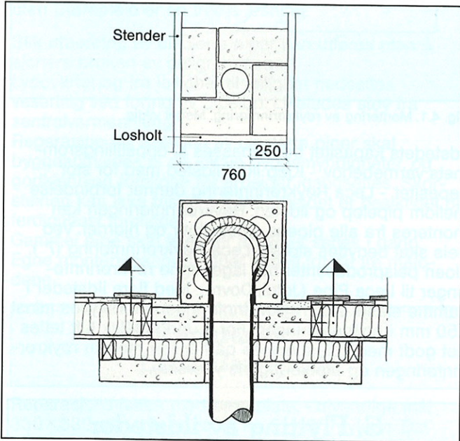
Fig. 1.6. Leca pipe kan monteres utvendig uten tilleggsisolering. Røykrør føres gjennom vegg og omslutes med Leca blokker som gir forskriftsmessig avstand til treverk. Innvendig 100 mm Leca blokk som brannmur.
