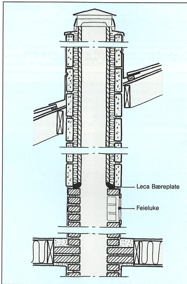
Fig. 2.2. Reparasjon med Leca Bæreplate.
