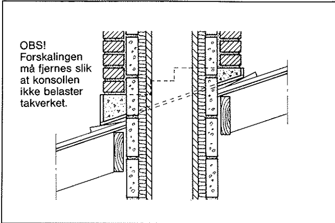
Fig. 2.1.2. Konsoll støpt på byggeplass.
