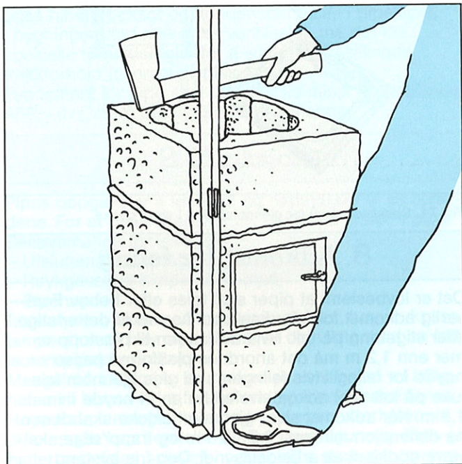
Fig. 1.2. Vatring og lodding er viktig!
