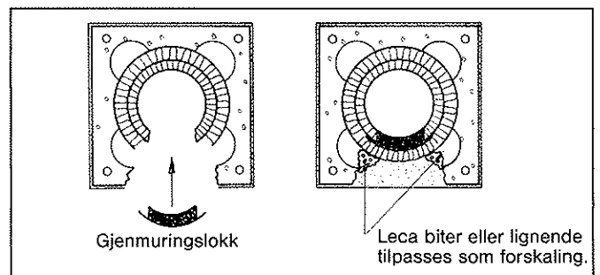
Fig. 5.1. Flytting av ildsteder.
