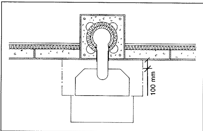
Fig. 5.2. Brannmurløsning.
