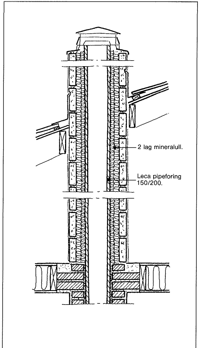
Fig. 4.1. Isolering/reparasjon.
