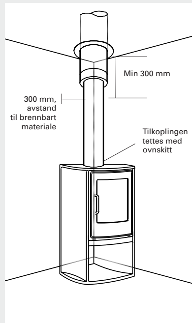
Eksempel på montering med uisolert startør.
