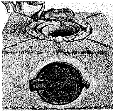
Fig. 2 Bunnen i feielukeelementet tildannes med mørtel — fall innover fra åpningen.
