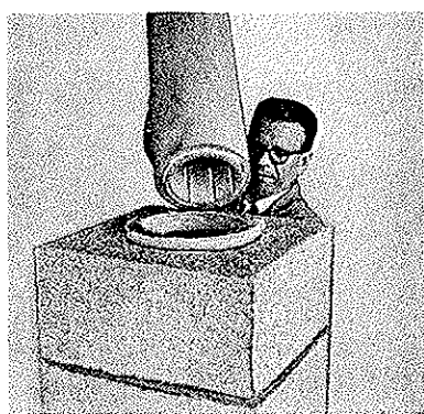
Fig. 5 Teglforingen (60 cm) settes på plass slik at skråkanten passer i den nedenfor.
