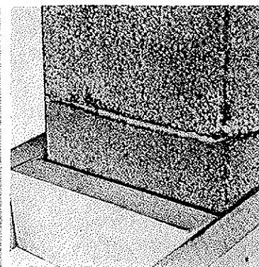
Fig. 8 Ved passering av bjelkelag skal det være noen mm klaring.
