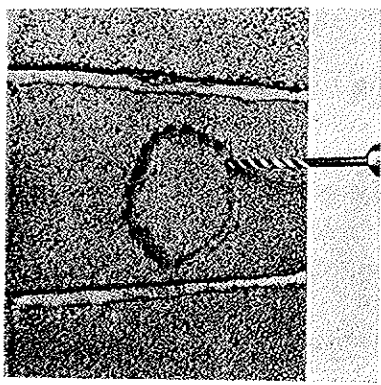
Fig. 9 Det merkes av for røykrørinnføring — bores en serie hull og Leca-biten meisles ut.
